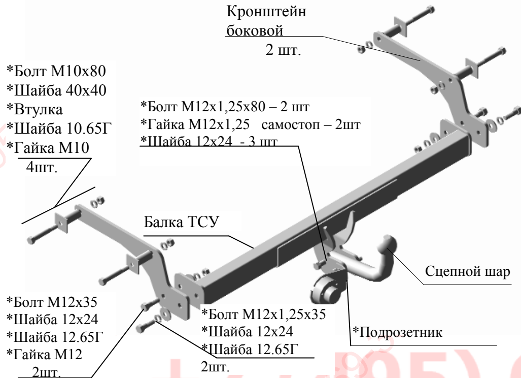
Рис.1 Тягово-сцепное устройство ТСУ 9010 Рено Логан.
